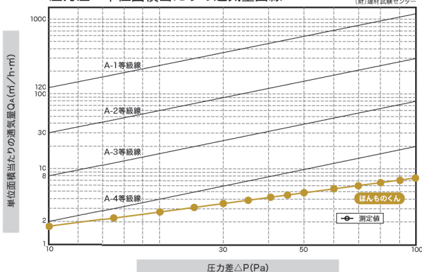
圧力差—単位面積当たりの通気量曲線
